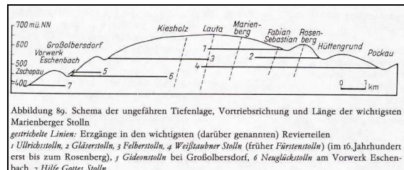
Abbildung 7: Die bedeutendsten Marienberger Stolln (Wagenbreth 1990)
